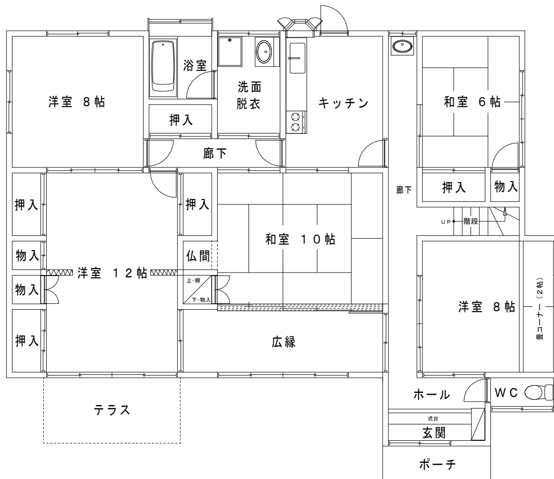
一階平面図
